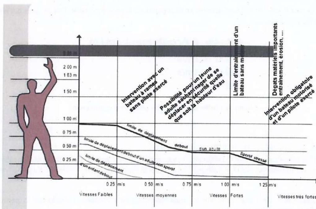
Figure 28 : Mobilité en terrain inondé en fonction de la vitesse et de la hauteur d'eau (Source : DDTM13)
