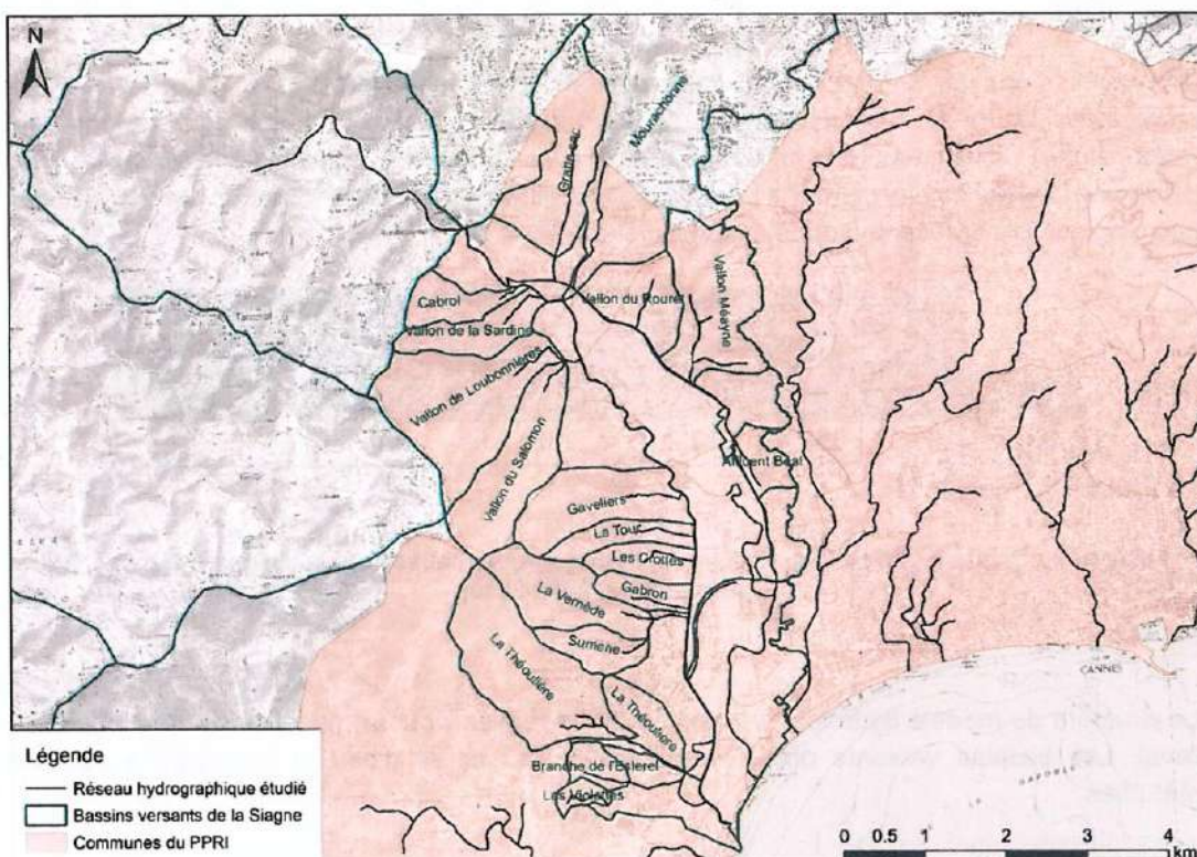
Figure 23 : Bassins versants de la Siagne faisant l'objet de l'analyse hydrologique
