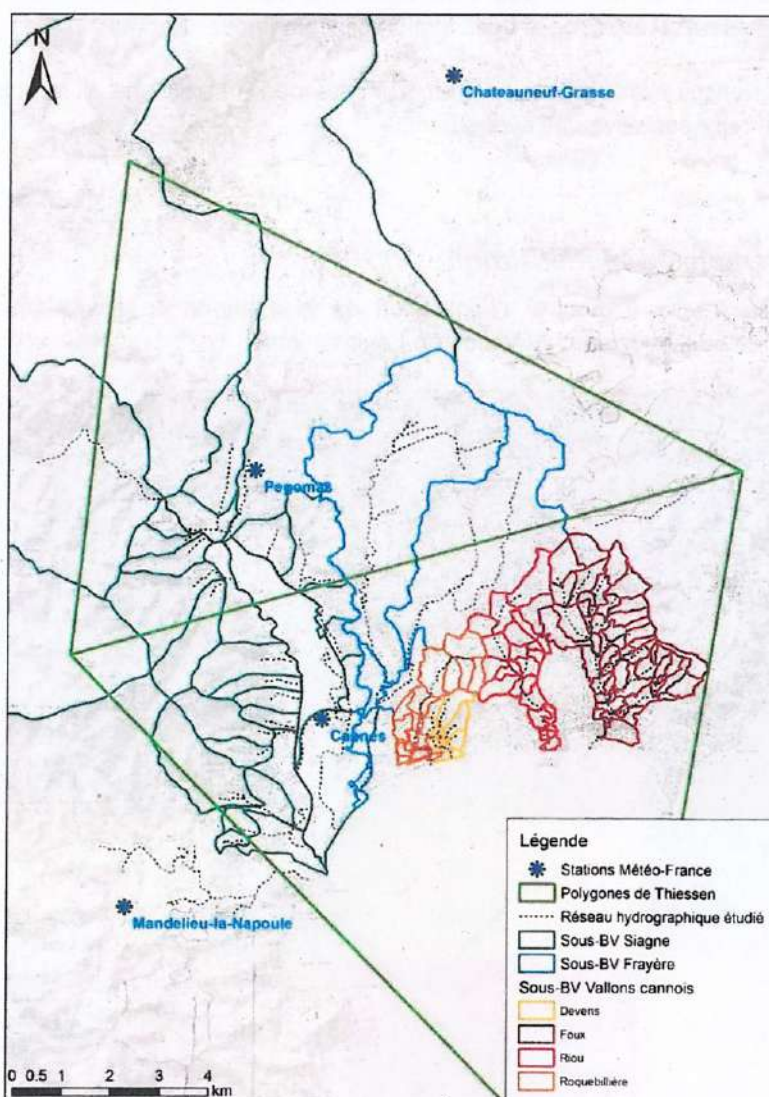
Figure 18 : Affectation des stations pluviométriques à chaque sous-bassin versant
