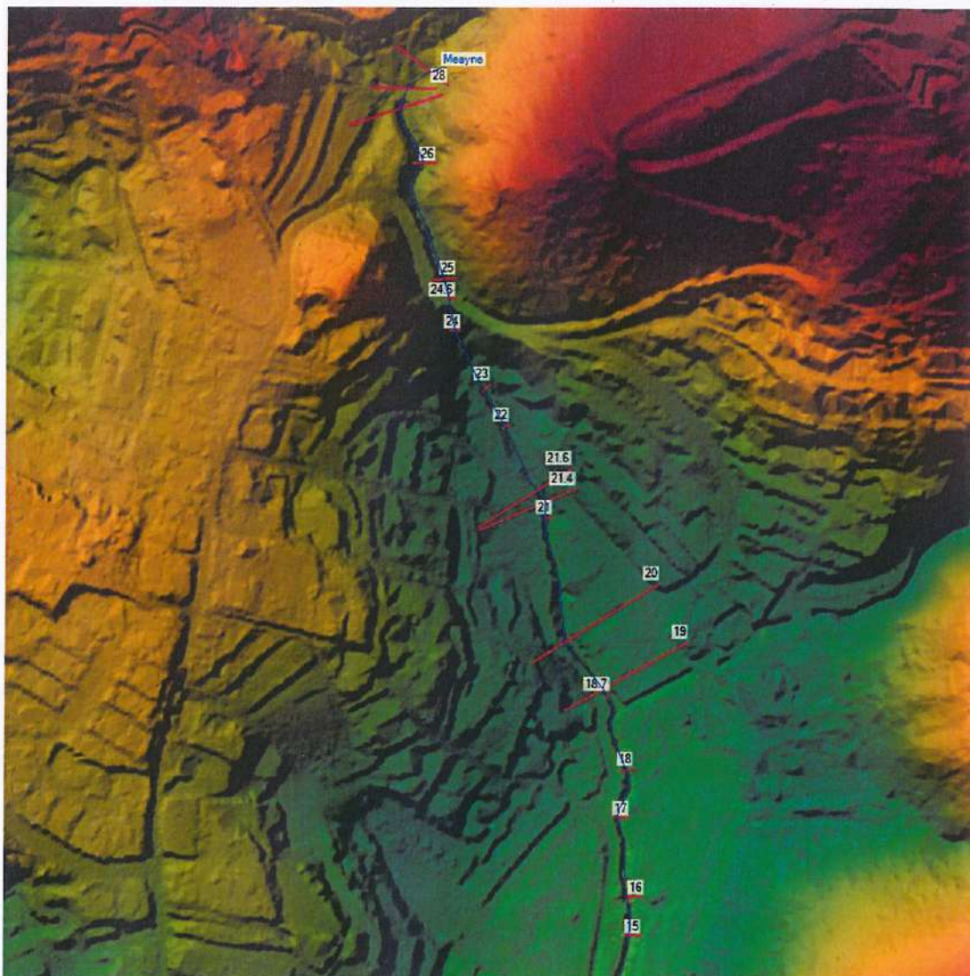
Figure 26 : Vue globale du modèle de la Meayne amont
