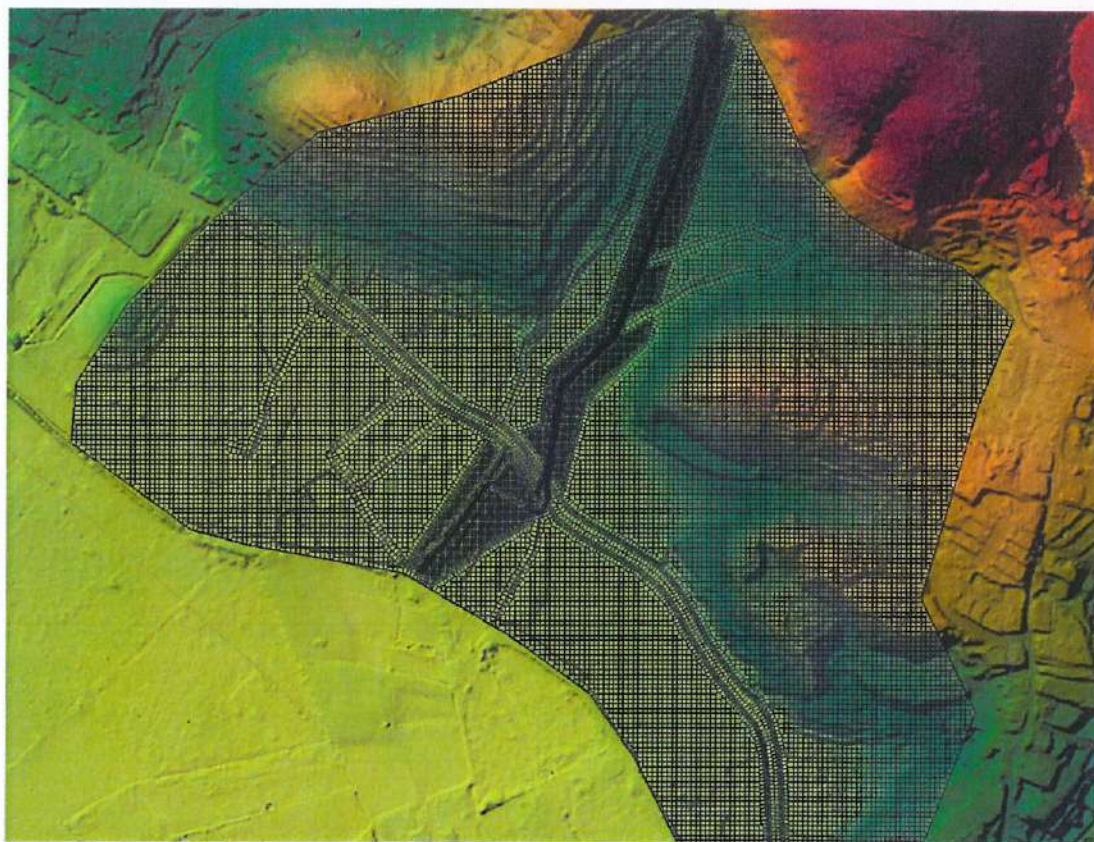
Figure 25 : Vue globale du modèle du Rouret
