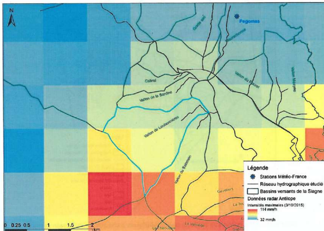
Figure 19 : Pluviométries radar sur le Vallon de Loubonnières et la station Météo-France de Pégomas
