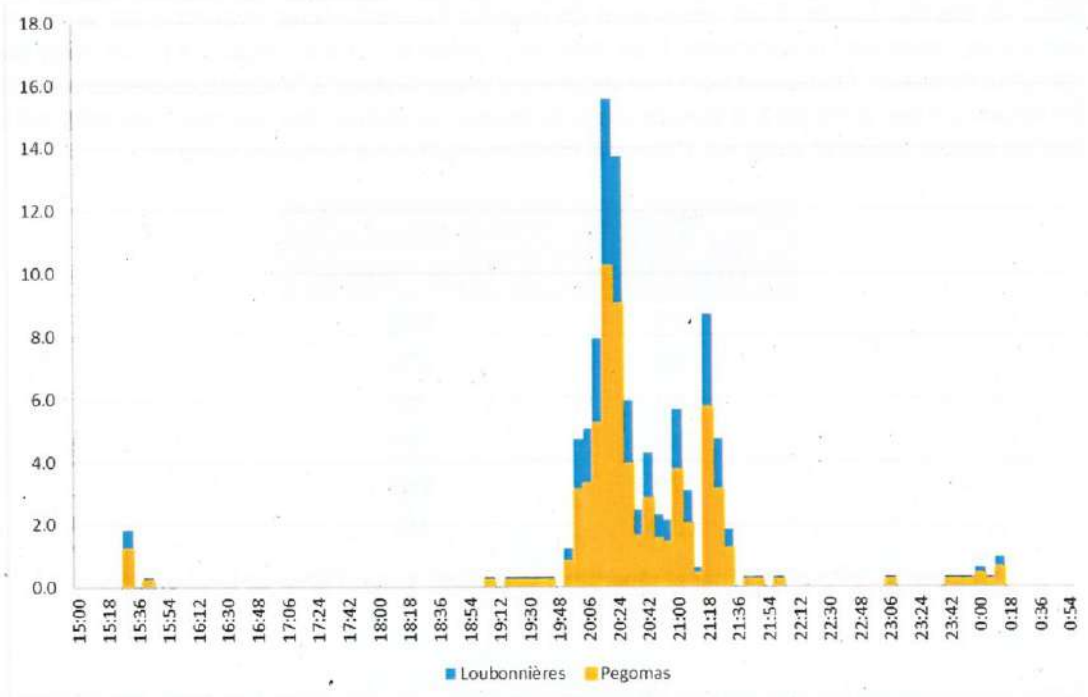
Figure 20 : Hyétogrammes du Vallon de Loubonnières et de la station de Pégomas
