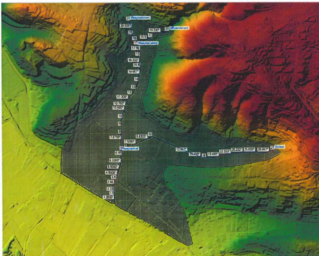
Figure 27 : Vue globale du modèle de la Meayne aval
