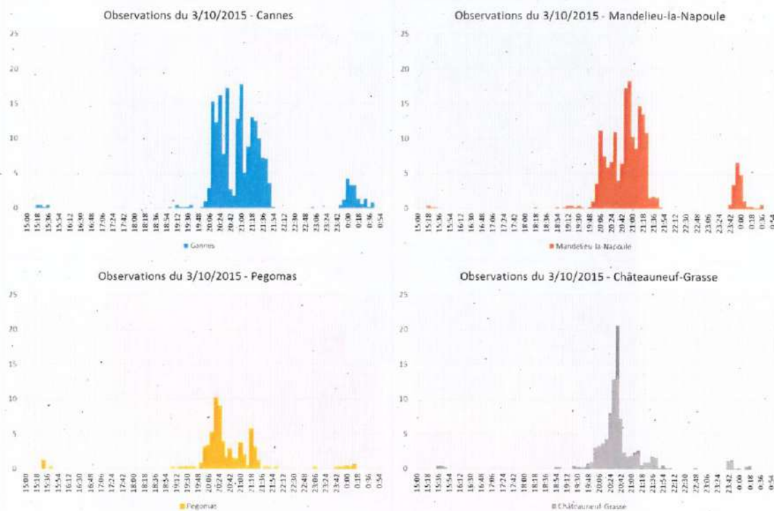
Figure 16 : Hyétogrammes du 3 octobre 2015, centrés sur l'évènement
