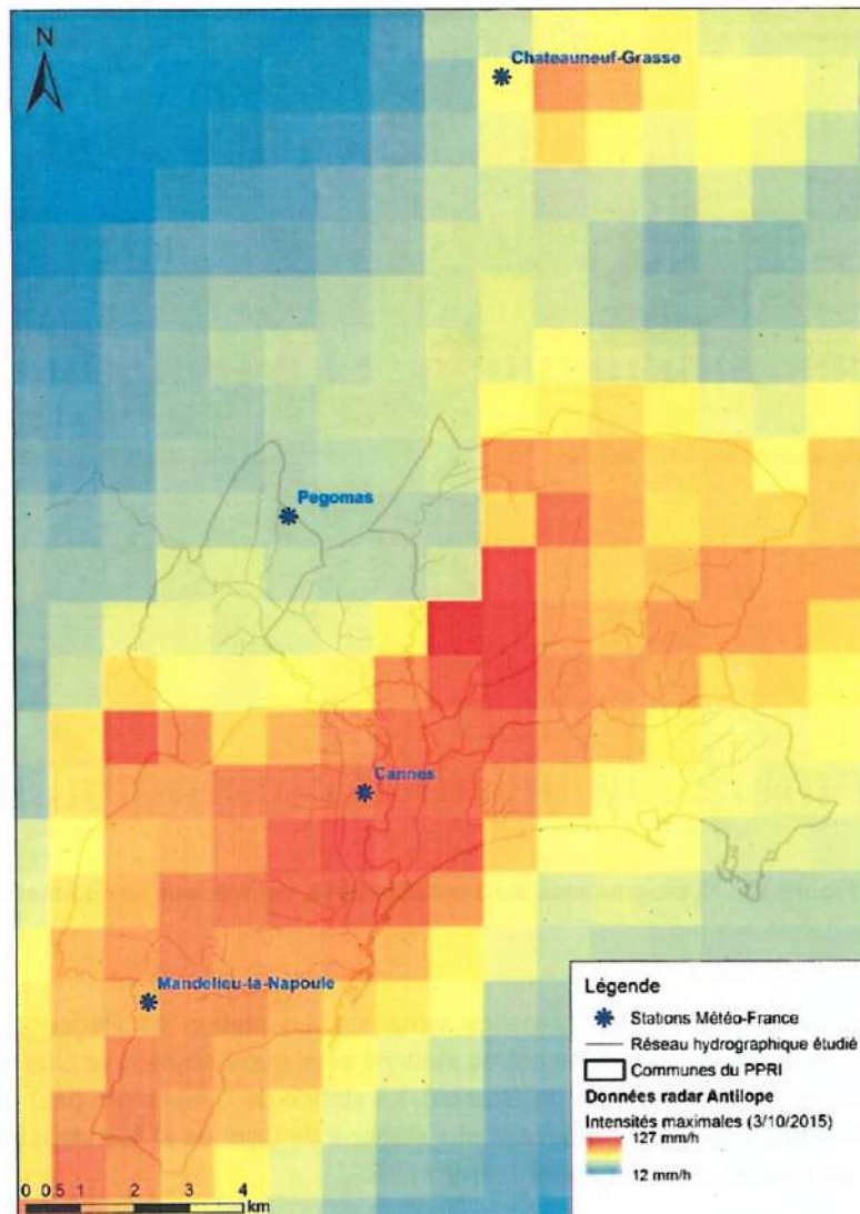
Figure 17 : Maximum des intensités radar Antilope pour l'évènement du 3/10/2015
