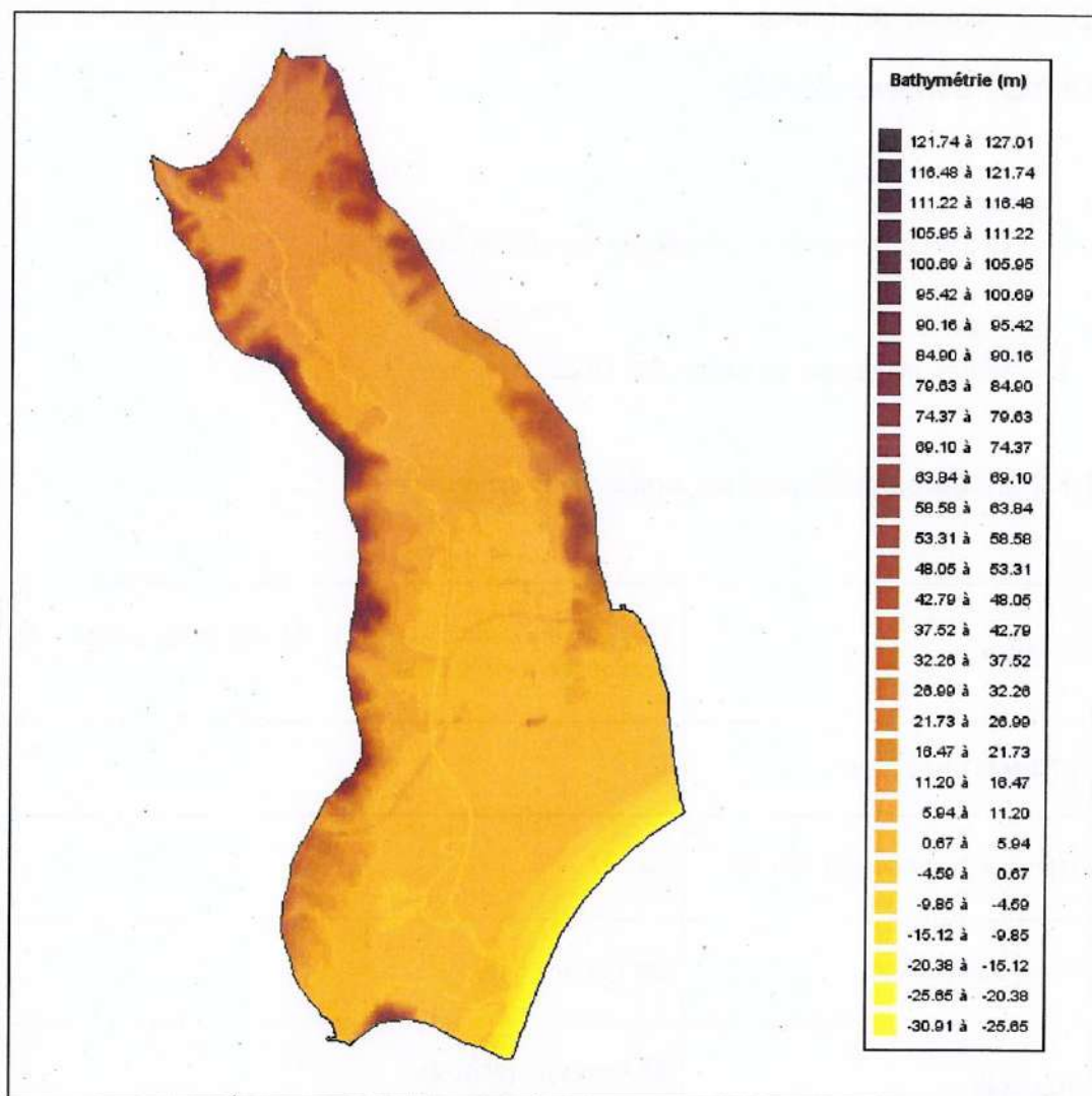
Figure 24 : Vue globale du modèle de la Siagne, du Béal, de la Vieille Siagne, du Gratte-Sac et de la Mourachonne
