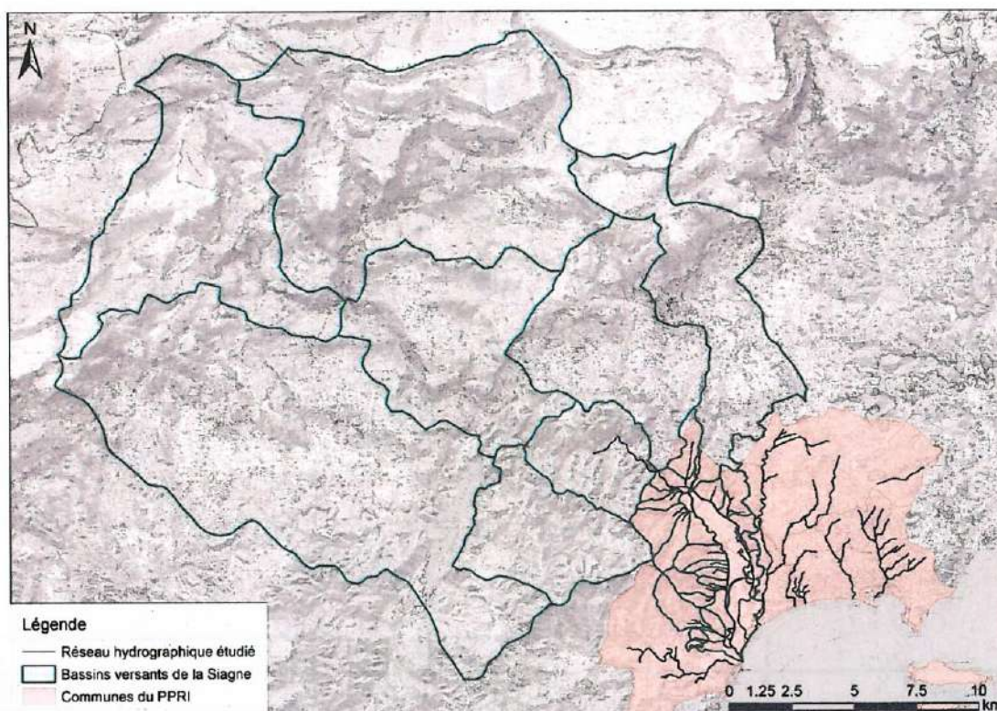
Figure 22 : Bassin versant de la Siagne et ses sous-bassins versants
